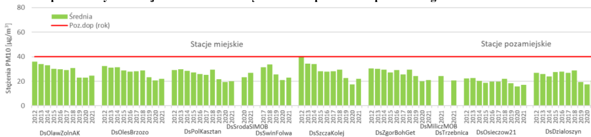
Wykres 1 Przebieg wartości średniej rocznej stężenia pyłu zawieszony PM10 na poszczególnych stanowiskach pomiarowych w województwie dolnośląskim na tle poziomu dopuszczalnego w latach 2012 - 2021
