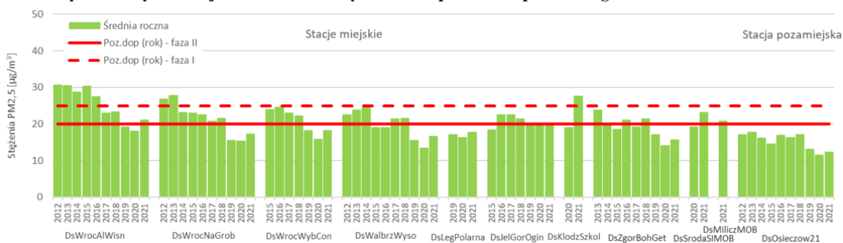
Wykres 2 Przebieg wartości stężenia średniego rocznego pyłu zawieszony PM2,5 na poszczególnych stanowiskach pomiarowych w województwie dolnośląskim na tle poziomu dopuszczalnego w latach 2012 – 2021
